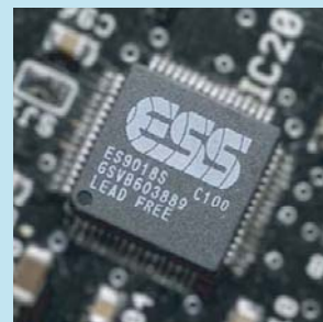
△ESS9018S (C-D1 デジタル基板)
